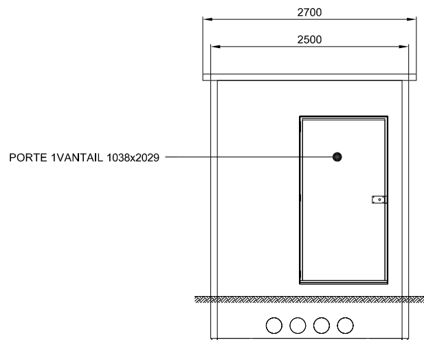
FACE AVANT
