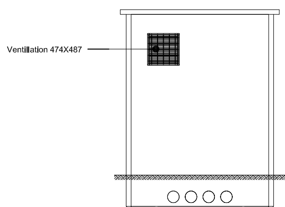
FACE ARRIERE
